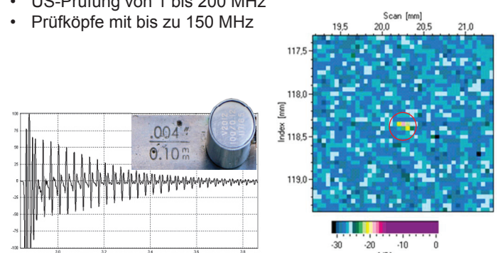
A-Bild einer 0,1 mm dicken Rasierklinge
