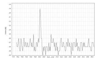
Echodynamikkurve einer 50 \mu\text{m} Flachbodenbohrung (C-Bild s.u.)
